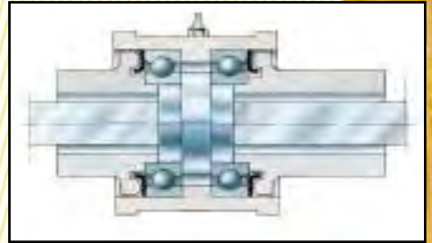
3800 – 4600 – 6400 mallien laakerointi
