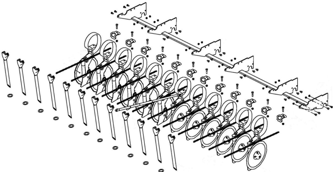
LASER-lannoitevantaisto
