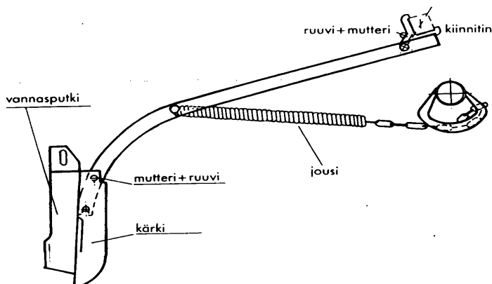
KUVA 36. Kylvövannas varsineen
