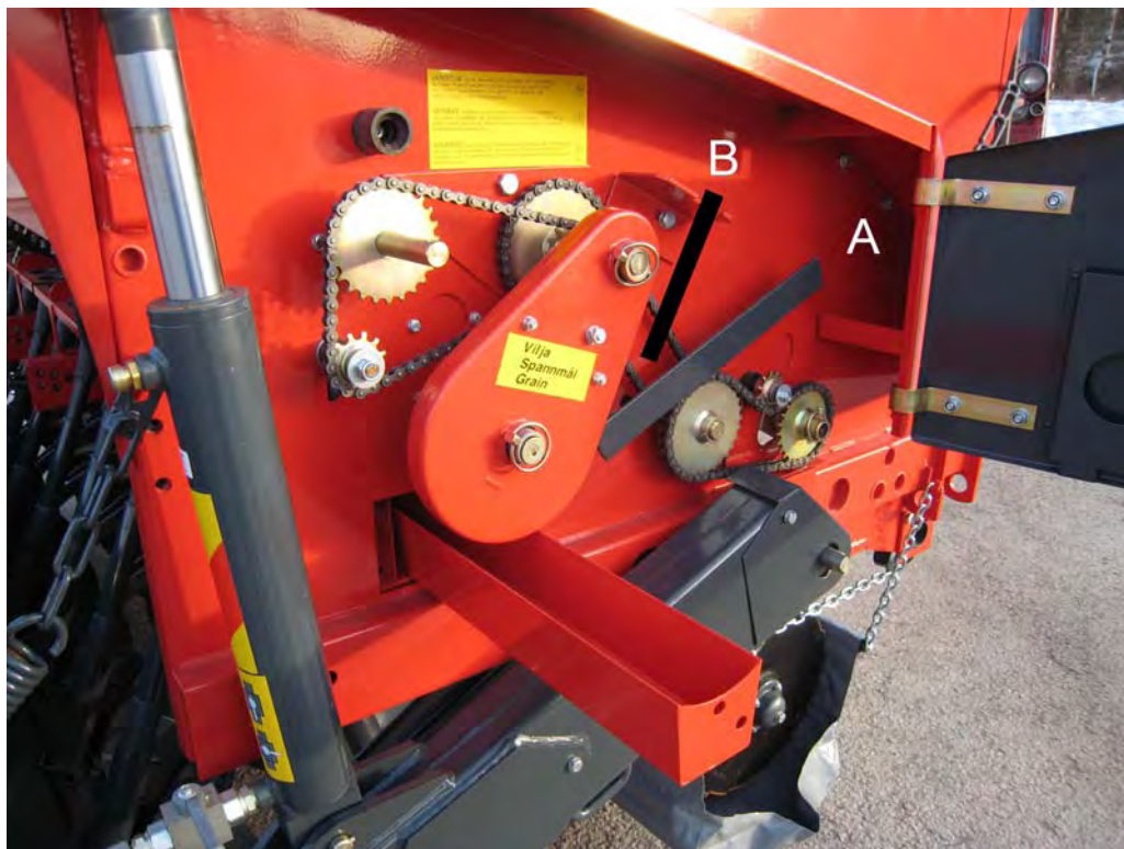
KUVA 23. Siemenpuolen kiertokoejärjestelmän käyttö
