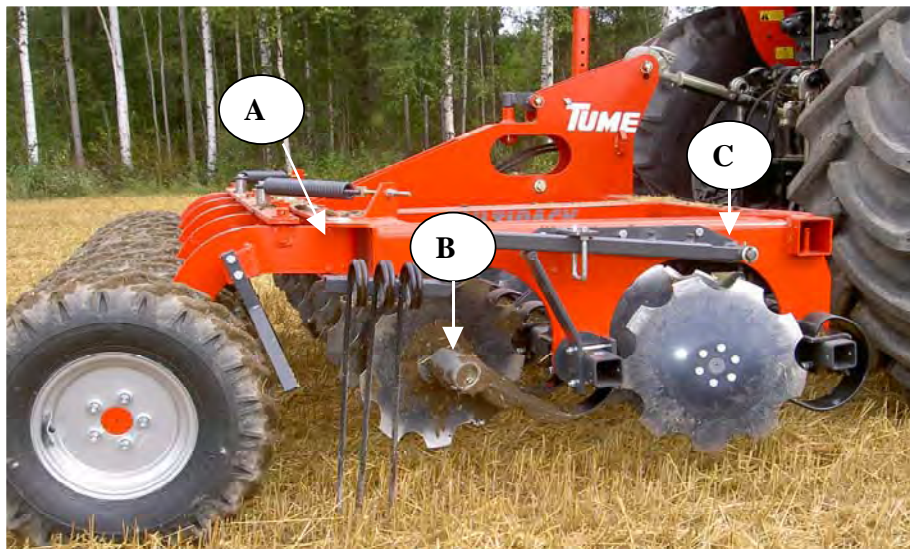
Kuva 12. Voitelukohteet A-C
