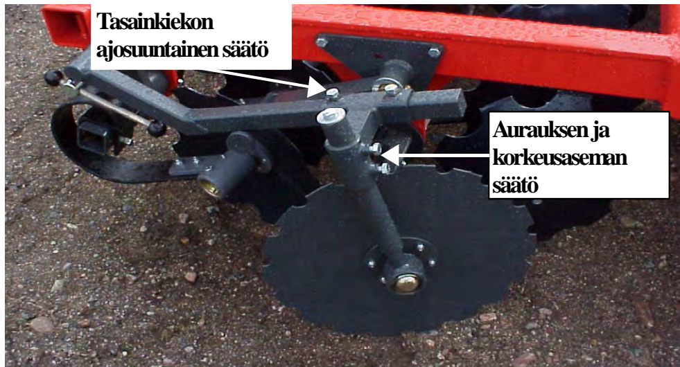
Kuva 7. Vasen vallintasain
