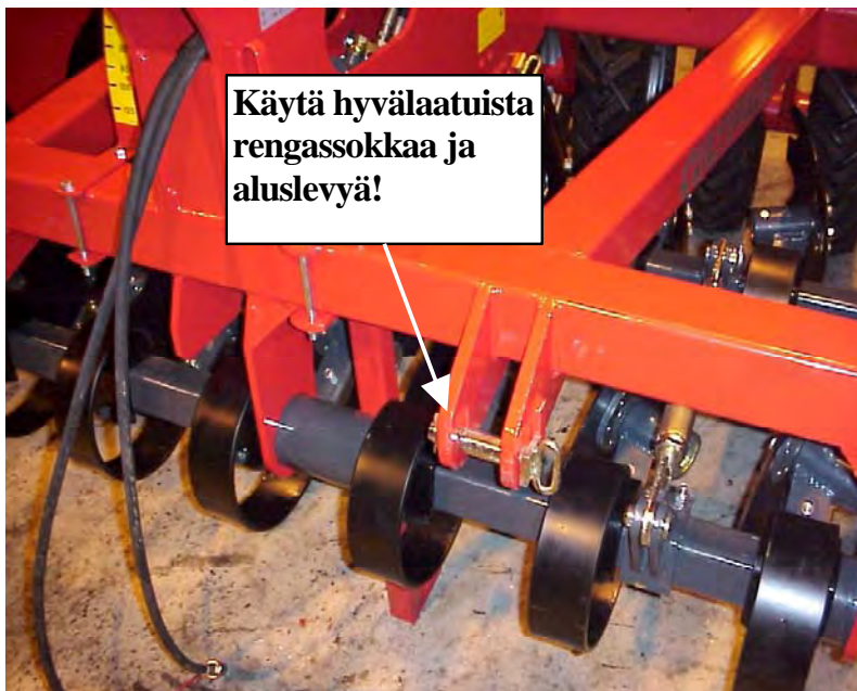
Kuva 1. Koska vetokorvissa on soikeat reiät, tulee rengassokan alla käyttää aluslevyä
