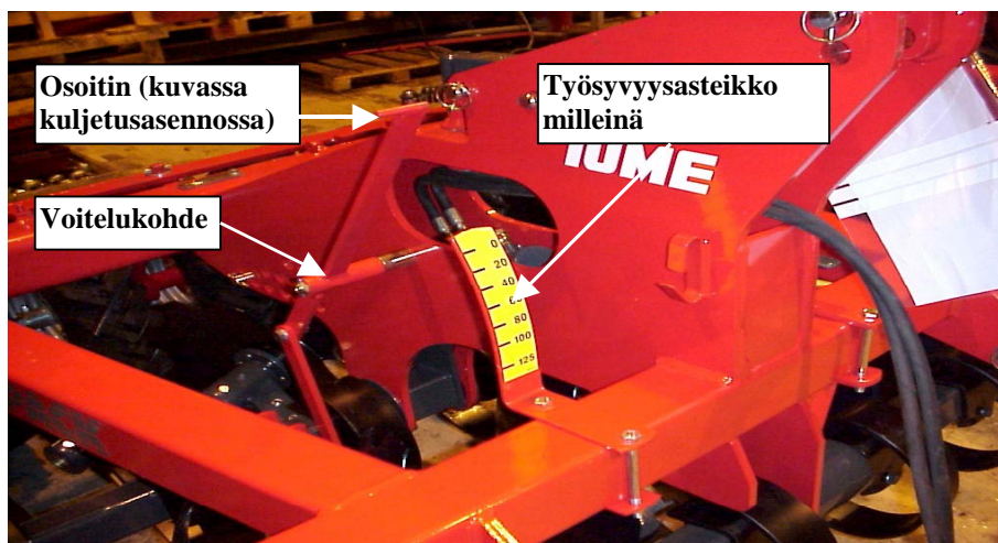
Kuva 4. Työsyvyyden osoitin ja asteikko
